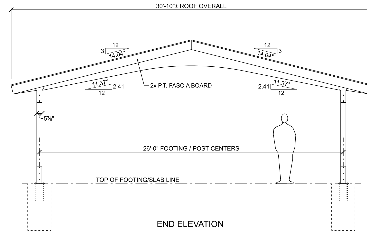
END ELEVATION
